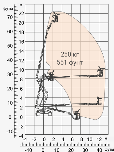
Диапазон перемещения
