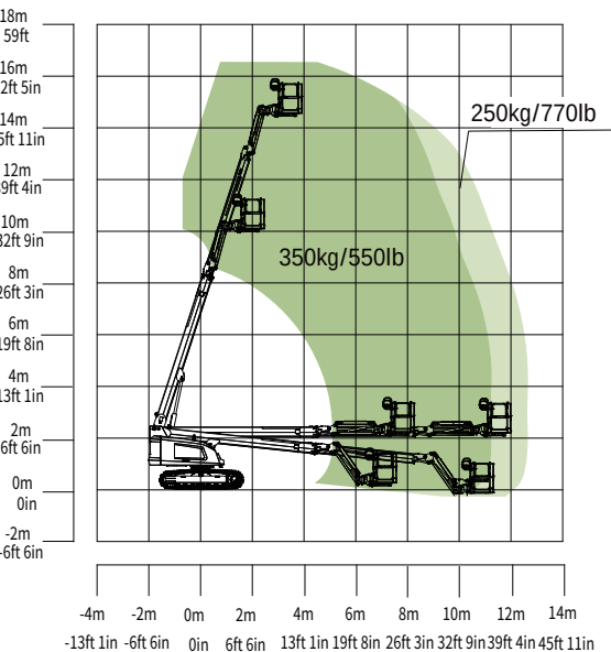
Диаопзон перемещения ZT14JC
